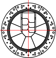
CAVE MAXI-RONDE Profondeur : 2,25m
