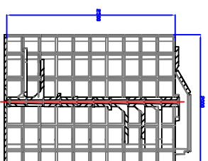
CAVE RONDE 2m Profondeur : 2,75m
